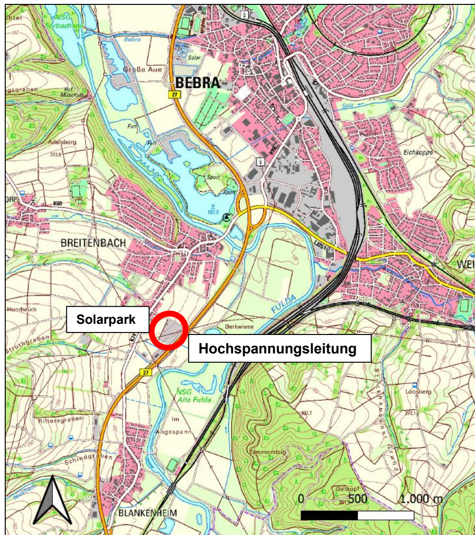
Lage der geplanten Photovoltaik-Freiflächenanlage
